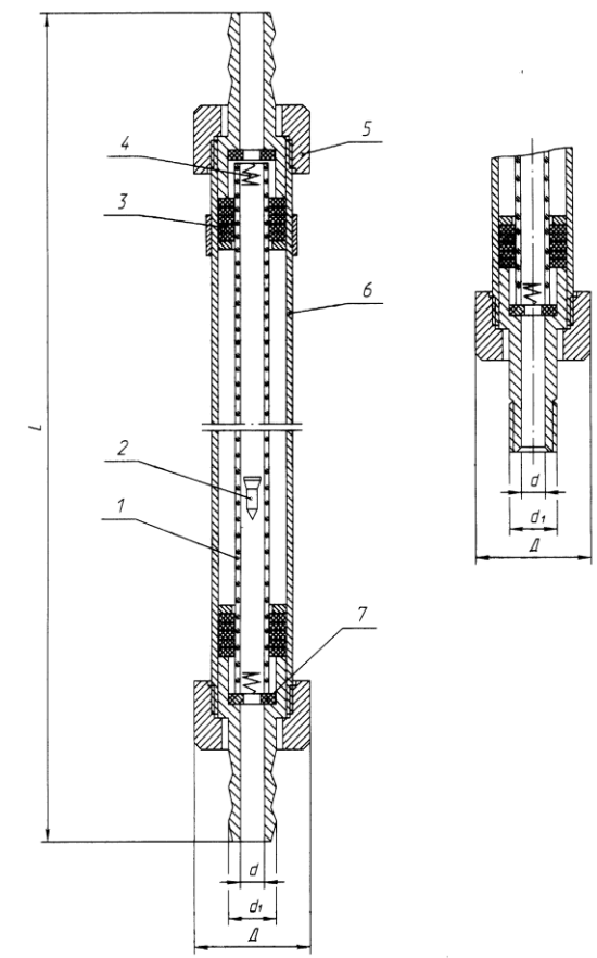
Размеры, мм
